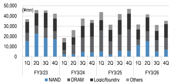
図表6: KOKUSAI Electricの装置売上
